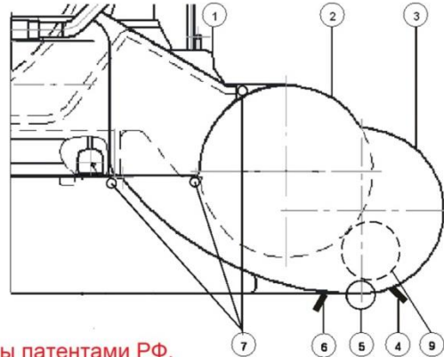
Схема Гибкого ограждения.
